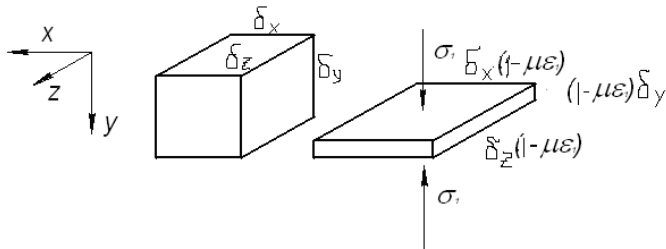
Рис. 1.3. Деформація під дією одноісного стиснення
