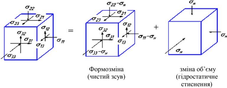
Рисунок 2.3 – Девіаторна та шарова складові тензора напружень
