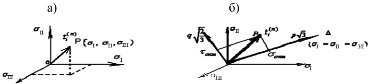
Рисунок 2.4 – а) простір головних напружень; б) осі гідростатичного тиску та девіатора
