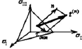
Рисунок 2.5 – Октаедрична площадка та нормаль n до неї
